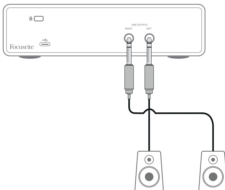
连接无源扬声器
