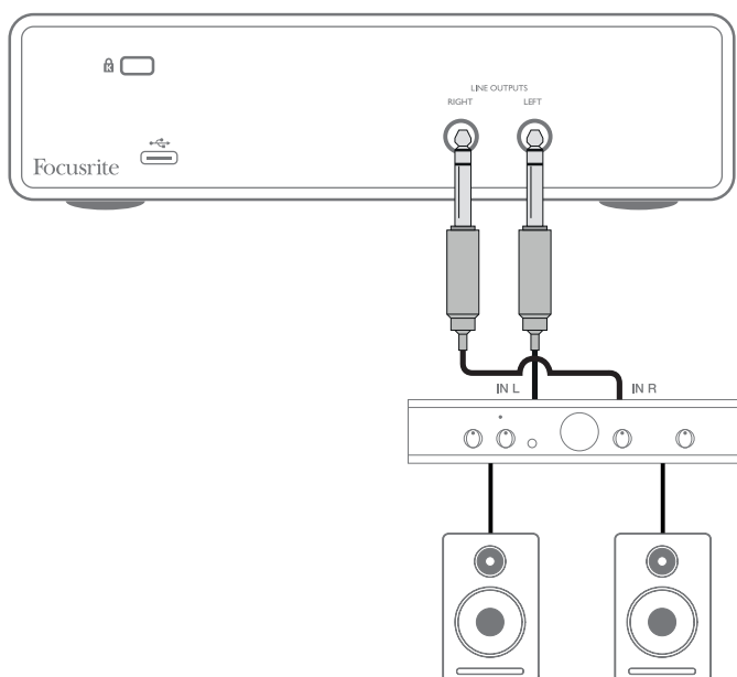
连接有源扬声器
