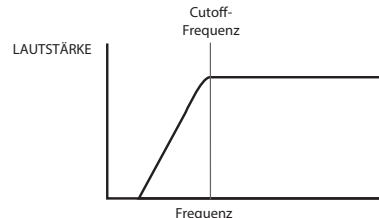
Hochpass 12 dB
